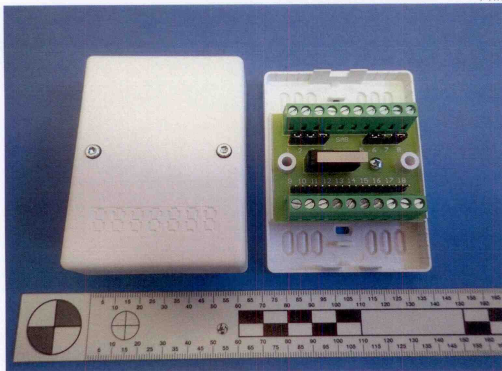
Modul montážních svorek MZ-2 L
